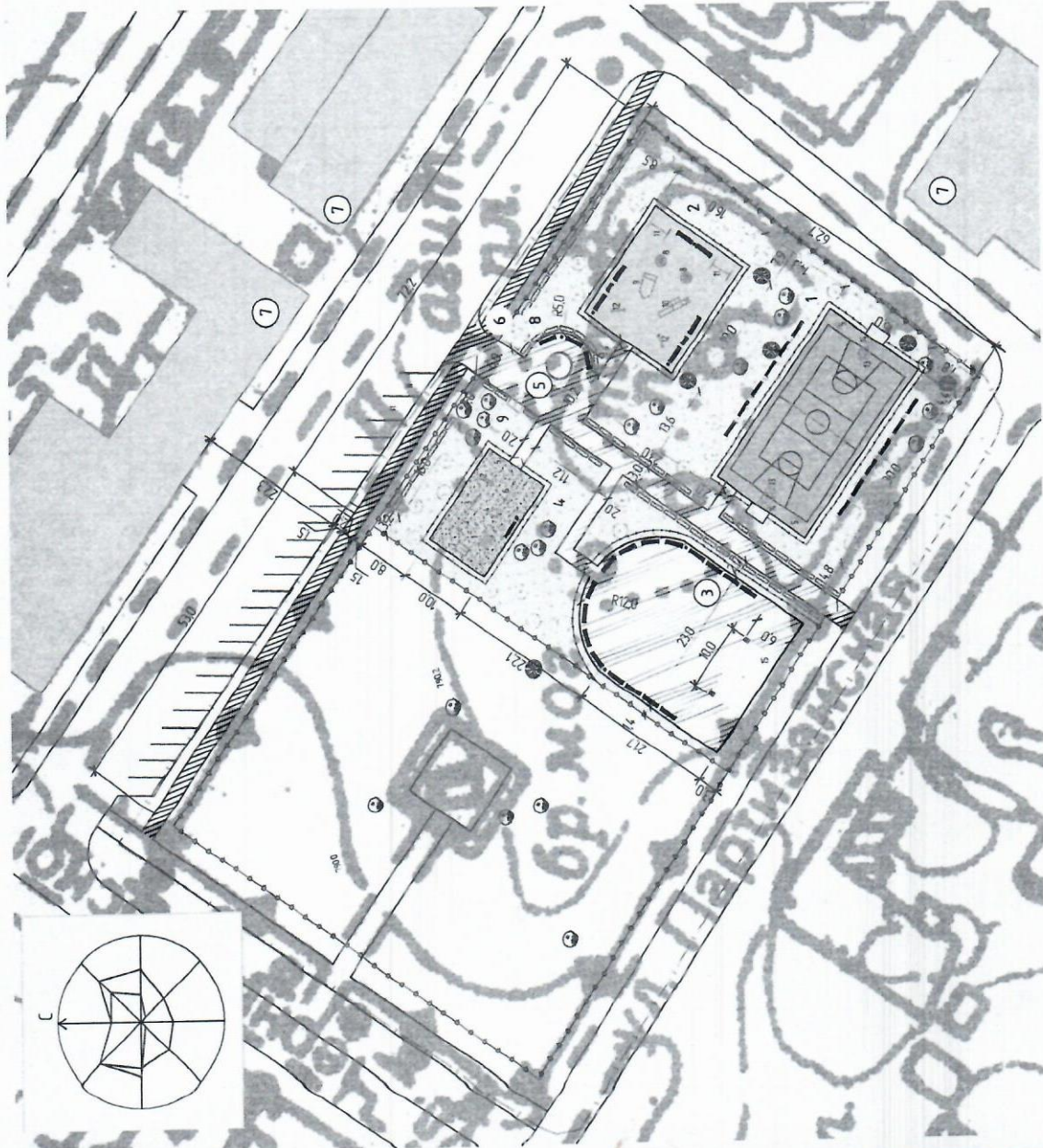
Схема планировочной организации земельного участка 1:500
